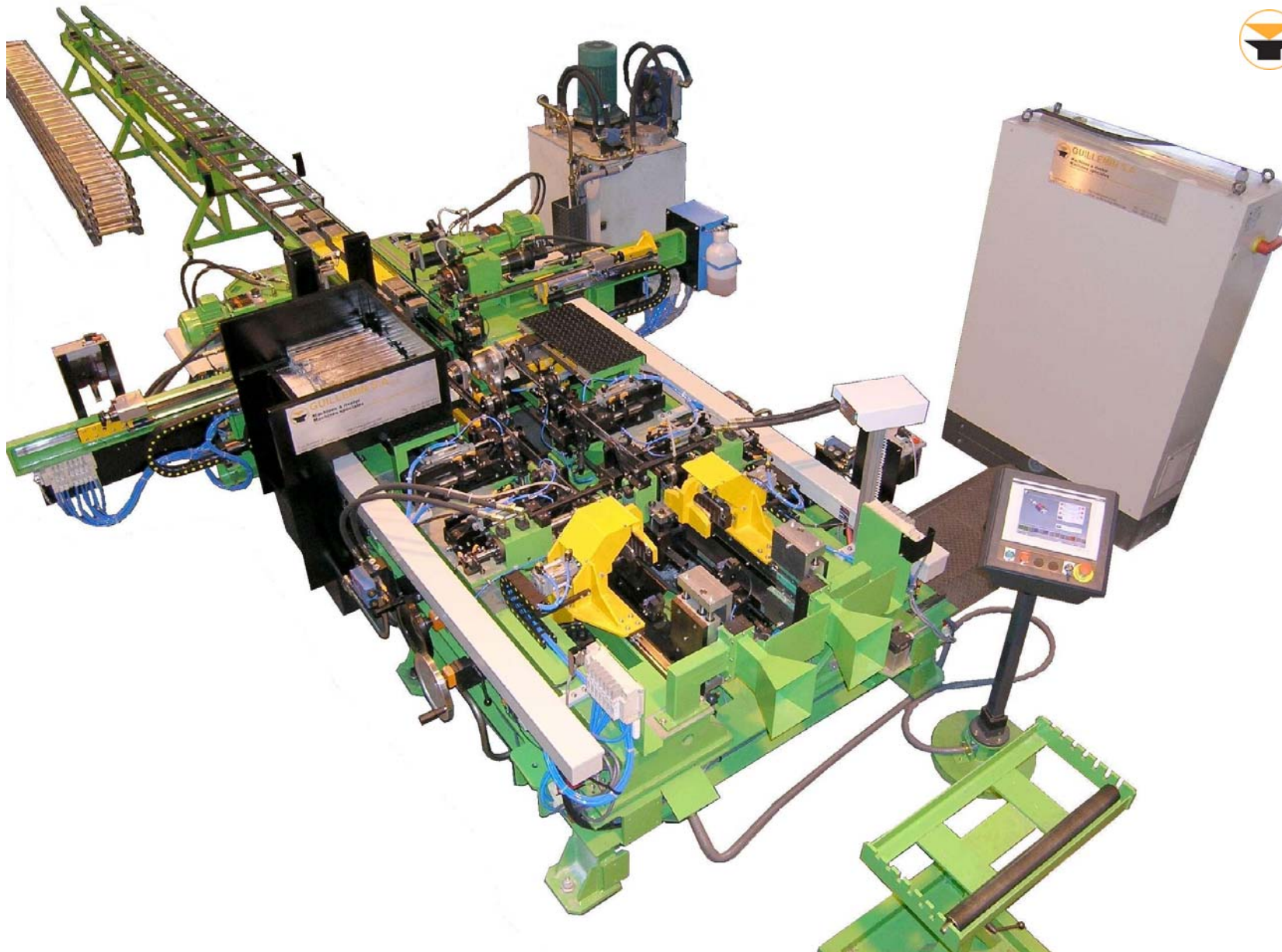
Vollautomatische Leiternfertigungsanlage P111 zur Herstellung von Aluminiumleitern mit festem Sprossenabstand, einstellbar für Breiten von 280—500 mm, mit den Funktionen Holme stanzen, Sprossen aus Magazin zuführen, Expandieren und Tauseln
